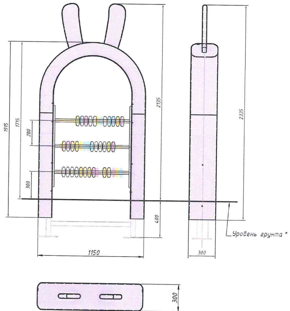
Рис. 3. Габариты изделия
