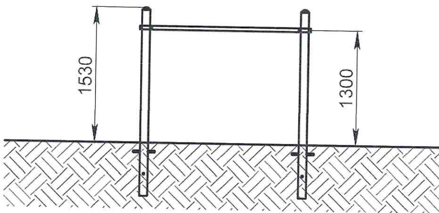
Рис. 3. Габариты изделия
