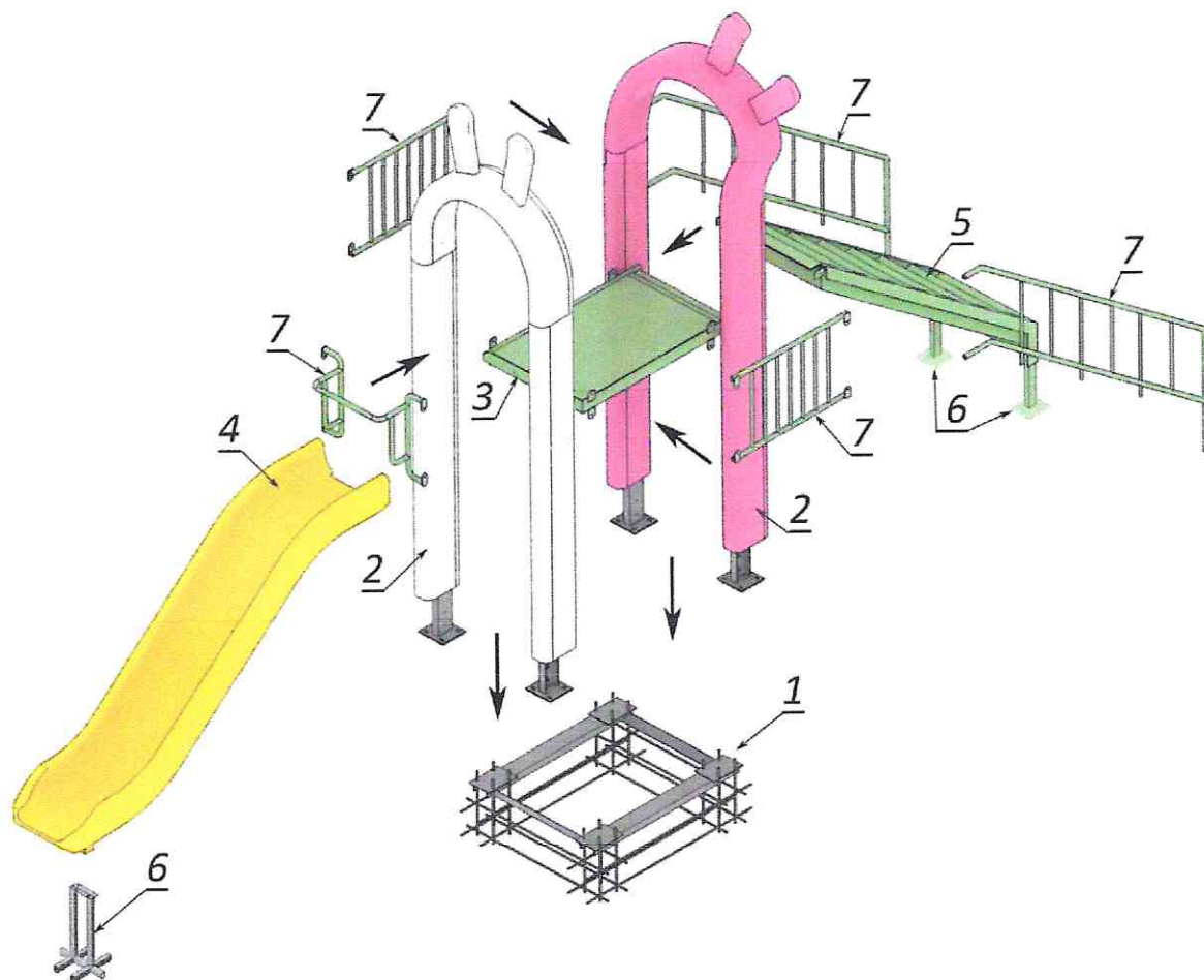
Рис. 4. Схема сборки изделия
