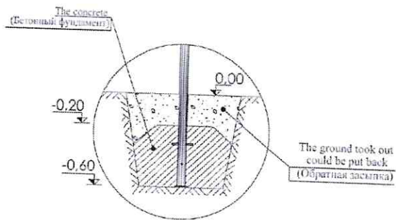
Рис. 4. Схема монтажа
