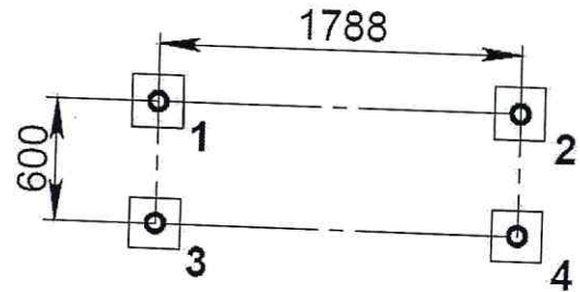
Рис. 5. Схема расположения фундаментов со стойками
